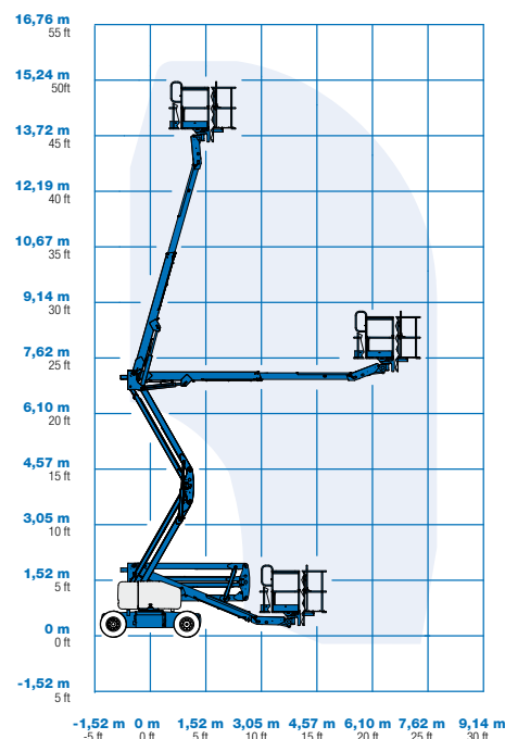
Diagramma di carico Z-45/25
