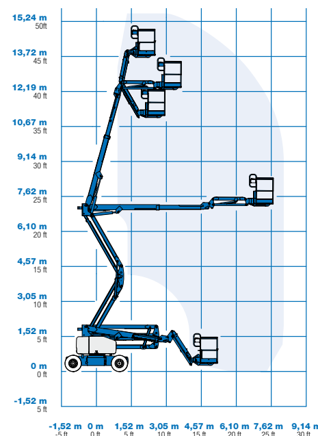
Diagramma di carico Z-45/25J
